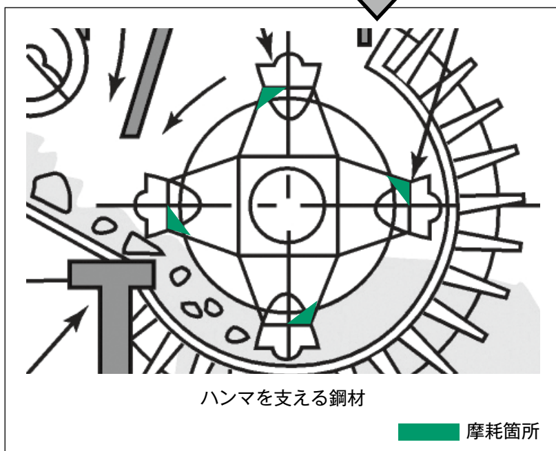
破砕機の断面図
